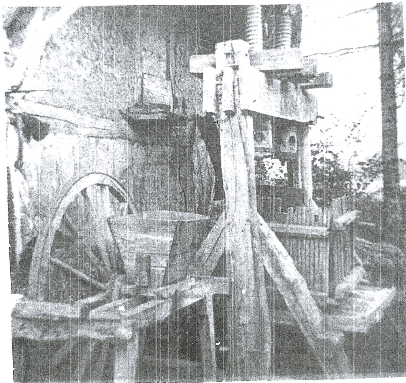
Pressoir à vis fin XVIIIe siècle
